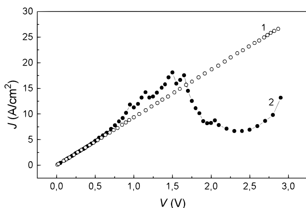
Рис. 1. Типові вольт-амперні характеристики зразків \text{In}_2\text{Se}_3 товщиною 600 мкм при T = 289 К: лінійна (крива 1), Z- і N- подібна (крива 2)
