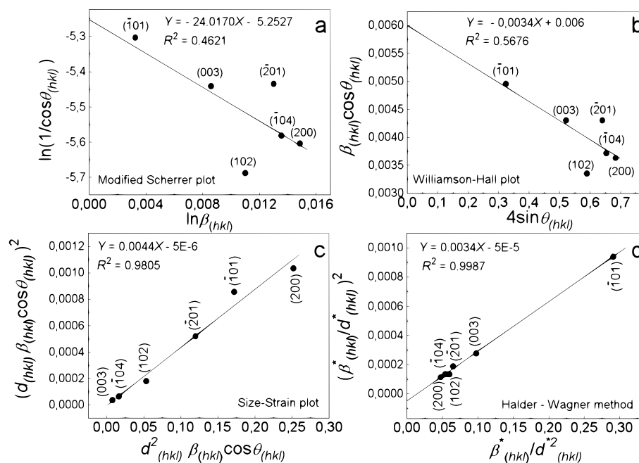
Рис. 3. Модифікована залежність Шеррера (а), а також залежності Вільямсона–Холла (b), розмірно-деформаційна (SSP) (c) і Холдера–Вагнера (d), побудовані для характеристики нанокристалітів \text{In}_6\text{Se}_6 у матриці шаруватого \alpha\text{-In}_2\text{Se}_3 . R^2 – величина достовірності апроксимації експериментальних даних (точки) відповідною залежністю (лінії)
