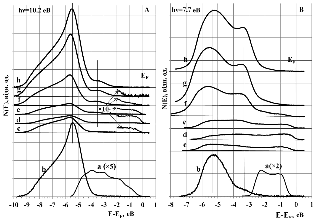
Рис. 2. ФЕС (А – h\nu = 10,2 еВ, В – h\nu = 7,7 еВ) фотокатода на різних етапах його випробування в одному із циклів досліджень: а – етапу атомарно чистої поверхні Si(100)-2 × 1; б – етапу типового початкового зразка; с – після нанесення \approx 0,5 МШ Gd; д – після нанесення \approx 1 МШ Gd; е, ф, г, h – етапи витримки системи з 1 МШ Gd у вакуумі протягом 1, 3, 6 та 12 діб, відповідно
