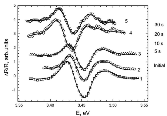
Рис. 1. Спектри ЕВ плівок GaN до і після мікрохвильової обробки. Символи – експериментальні дані, криві – результати теоретичної підгонки: 1 – вихідний зразок; 2 – впродовж 5 секунд; 3 – впродовж 10 секунд; 4 – впродовж 20 секунд; 5 – впродовж 30 секунд
