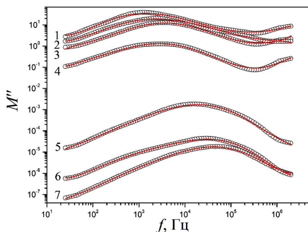
Рис. 3. Залежність уявної частини електричного модуля від частоти для систем на основі матриці ПМК (1), яка містить: 0,1% (2); 0,25% (3); 0,5% (4); 0,75% (5); 1% (6); 1,5% (7) ВНТ. Порожні кола – експериментальні дані, суцільна лінія – апроксимація емпіричної функцією Гавриляка–Негами
