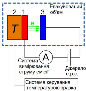
Рис. 6. Блок-схема експерименту з вимірювання роботи виходу методом термоелектронної емісії: 1 – досліджуванний зразок; 2 – нагрівач, що підтримує наперед задану температуру зразка; 3 – анод
