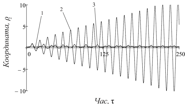
Рис. 3. Траєкторія руху мікрочастинки вздовж осі z у кровотоку: 1 – стаціонарна точка траєкторії, побудована за аналітичним виразом (13), 2 – траєкторія побудована на результаті чисельного розрахунку рівняння (15) при невиконанні умови (14), 3 – траєкторія, побудована при виконанні умови (14) на результаті чисельного розрахунку рівняння (15). (Координати вказані в безрозмірних величинах)
