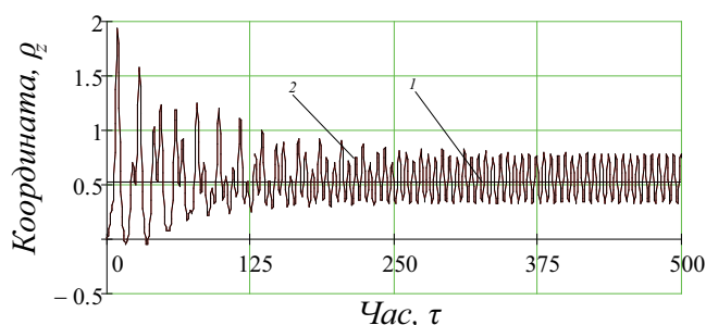
Рис. 2. Траєкторія руху мікрочастинки вздовж осі z у водяно-му потоці: 1 – стаціонарна точка траєкторії, побудована за аналітичним виразом (13), 2 – траєкторія, побудована на результаті чисельного розрахунку рівняння (14). (Координати вказані в безрозмірних величинах)
