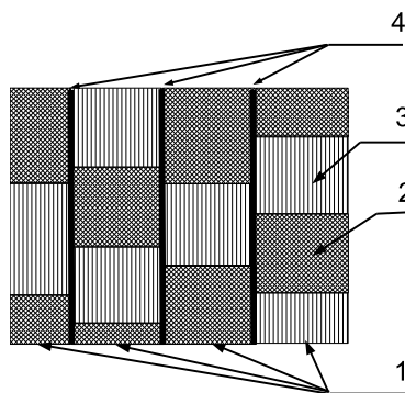
Рис. 1. Фібрилярний структурний рівень волокна: 1 – фібрили, 2 – неупорядковані внутрішньофібрилярні області, 3 – впорядковані внутрішньофібрилярні області, 4 – неупорядковані міжфібрилярні області
