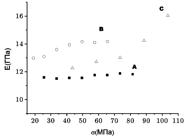
Рис. 2. Залежність модуля пружності від навантаження E(\epsilon) для зразків: А – фіброїнове волокно, отримане безпосередньо із залоз шовкопряда, В – фіброїнове волокно, отримане із залоз шовкопряда і оброблене лужним розчином, С – фіброїнове волокно, отримане з кокона шовкопряда
