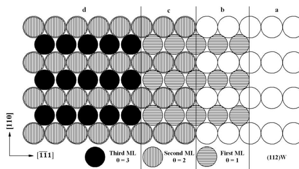
Рис. 1. Модель грані (112)W з трьома адсорбованими моношарами Cu. (a) – чиста грань, (b, c, d) – відповідно перший, другий і третій геометричні моношари Cu (ML). Фізичний моношар утворюють перші два геометричні (зона c)
