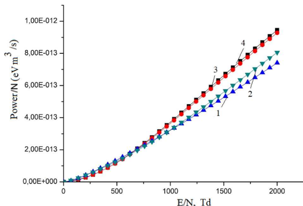
Рис. 10. Залежність питомої потужності втрат розряду на непружні процеси зіткнень електронів з атомами аргону, алюмінію і міді від приведеної напруженості електричного поля в плазмі газо-парових сумішей: 1 – Ar–Al–Cu = 13300 Па : 10000 Па : 10000 Па при загальному тиску 33300 Па, 2 – Ar–Al–Cu = 101000 Па : 10000 Па : 10000 Па при загальному тиску 121000 Па, 3 – Ar–Al–Cu = 13300 Па : 100 Па : 100 Па при загальному тиску 13500 Па, 4 – Ar–Al–Cu = 101000 : 100 : 100 при загальному тиску 101200 Па
