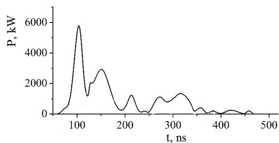
Рис. 1. Імпульсна потужність перенапруженого наносекундного розряду між двома електродами, виготовленими з халькопіриту при: p(\text{Ar}) = 101 кПа
