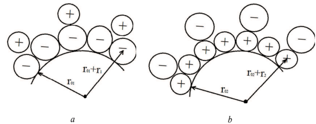
Рис. 5. Елемент ядра сферичної міцели. ПВІ є SO_4^{2-} (а), ПВІ є Ca^{2+} (б)
