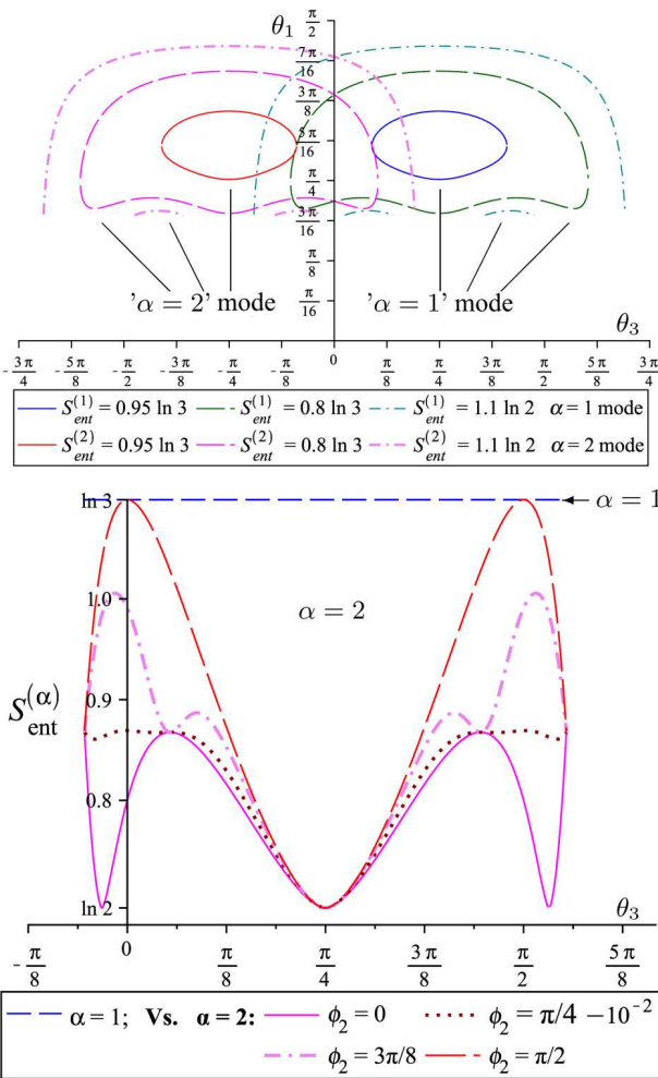
Рис. 2. Зверху: еквіентропійні криві ( S_{ent}^{(\alpha)} = \text{const} ) як функції кутів \theta_1 і \theta_3 при фіксованому \theta_3^{\mp} = \frac{\pi}{3} . Знизу: Ентропія заплутаності S_{ent}^{(2)}(\theta_3, \phi_2) для коферміона в \alpha = 2 моді при фіксованій ентропії заплутаності S_{ent}^{(1)} = \max = \ln 3 для \alpha = 1 коферміона
