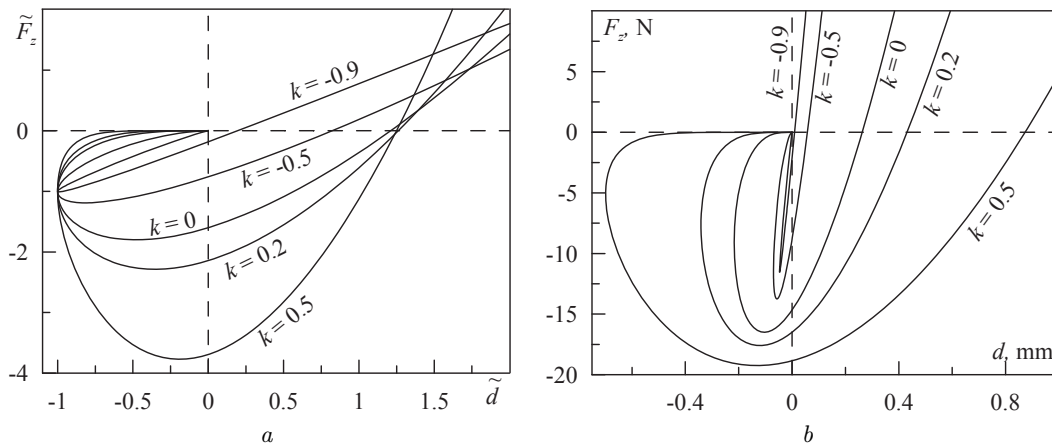
Рис. 2. Залежності пружної сили \tilde{F}_z від глибини інденування \tilde{d} для нормального адгезійного контакту. Криві відповідають аналітичному розв'язку (17) і (18) для фіксованих значень параметра k (a); залежності, які відповідають кривим на рис. 2, а у розмірному вигляді, при параметрах \Delta\gamma = 0,7 Дж/м 2 , c_0 = 1 м, R = 5 м, E = 10^6 Па, \nu = 0,3 (b)
