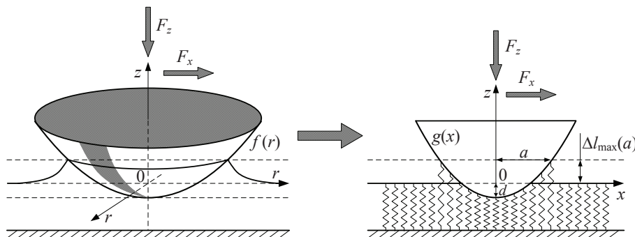
Рис. 1. MDR трансформування оригінального тривимірного профілю f(r) у одновимірний g(x) і заміна пружного напівпростору пружною основою із не взаємодіючих пружин. При наявності нормальної і тангенціальної сил і адгезії пружини основи будуть зсуватися одночасно у нормальному і тангенціальному напрямках. На рис. 1 проілюстровано лише нормальний рух індентора і стискання пружин у цьому напрямку
