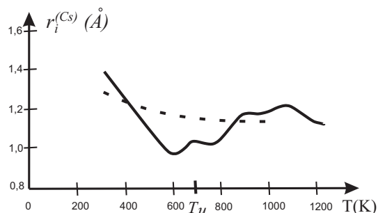
Рис. 2. Температурна залежність r_i^{(Cs)} : суцільна лінія відповідає i = D , штрихова – i = \text{eff} . Символ T_u позначає положення верхньої границі температурного інтервалу фізично коректних значень MRT для рідкого Cs
