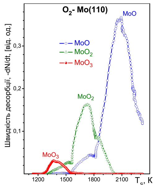
Рис. 6. Швидкість випаровування оксидів від температури підкладки T_S в умовах постійного потоку кисню F = 4 \cdot 10^{12} мол/(см 2 ·с) на поверхні Mo(110). Швидкість лінійного нагріву зразка \chi = 20 К·с -1
