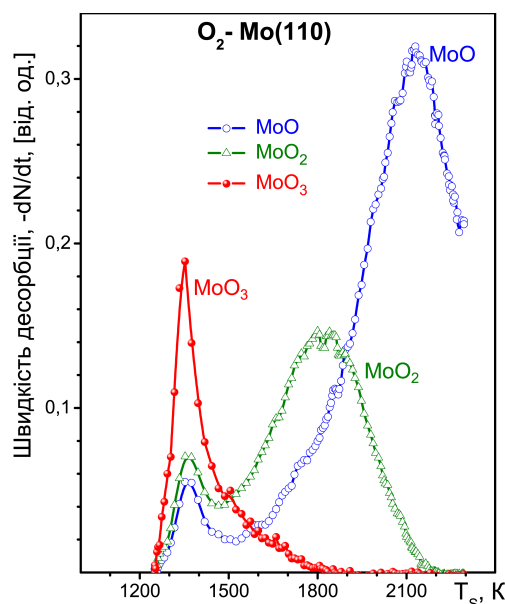
Рис. 7. Швидкість випаровування оксидів від температури підкладки T_S в умовах постійного потоку кисню F = 8 \cdot 10^{14} мол/(см 2 ·с) на поверхню Мо(110). Швидкість лінійного нагріву зразка \chi = 20 К·с -1
