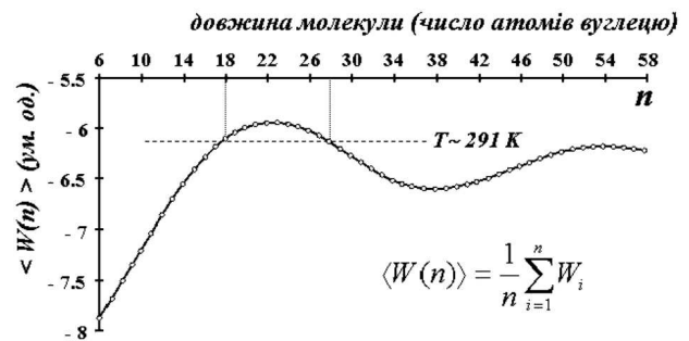
Рис. 7. Залежність середньої енергії взаємодії \text{CH}_2 -груп, \langle W(n) \rangle , молекул n -алканів, адсорбованих на Au(111). Розрахунок проведений для інтервалу 6 \leq n \leq 58 ( n – парні). Пунктирна пряма відтворює ділянку кривої \langle W(n) \rangle , що відповідає інтервалу нестабільності ( 18 \leq n \leq 26 )
