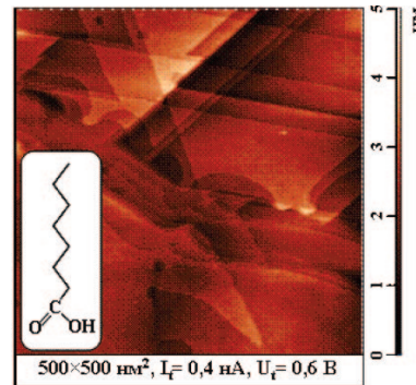
Рис. 8. СТМ-зображення моношару n -октанової кислоти \text{CH}_3-(\text{CH}_2)_6-\text{COOH} на поверхні Au(111) (субмікронний масштаб). На вставці – структурна формула n -октанової кислоти
