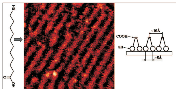
Рис. 10. СТМ-зображення моношару тиолізованої n -додеканової кислоти на Au(111). Спостерігається рядкова структура з подвійним періодом. Параметри сканування: 10 \times 10 \text{ нм}^2 , I_t = 0,5 \text{ нА} , U_t = 500 \text{ мВ} . Праворуч – схематичне пояснення структури пакування. Подвійний період зумовлено асоціацією COOH-груп молекул сусідніх рядків
