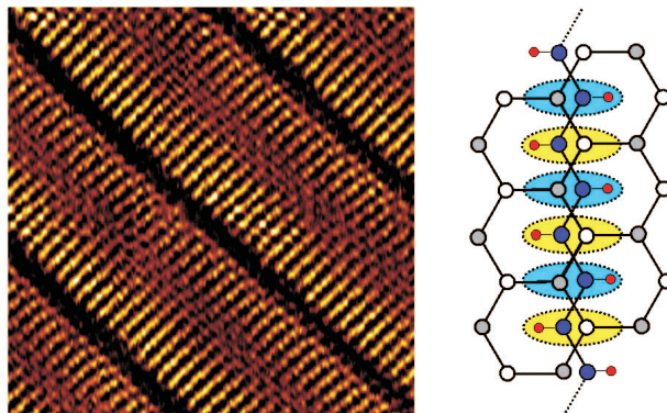
Рис. 3. СТМ-зображення моношару n - C_{36}H_{74} на графіті (ліворуч). Параметри тунелювання: 21 \times 21 \text{ nm}^2 ; U_t = 100 \text{ мВ} ; I_t = 0,1 \text{ нА} . Праворуч – схематична модель, яка пояснює підсилення СТМ-контрасту кожної другої CH_2 -групи алкільного ланцюга, адсорбованого на графіті (пояснення див. у тексті)
