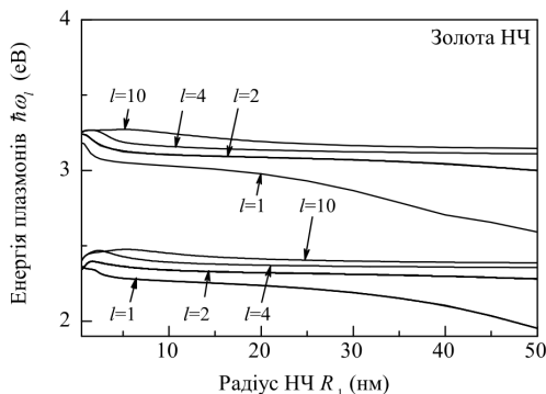
Рис. 4. Енергії інтерфейсних плазмонів золотої НЧ з різними орбітальними числами l залежно від радіуса НЧ
