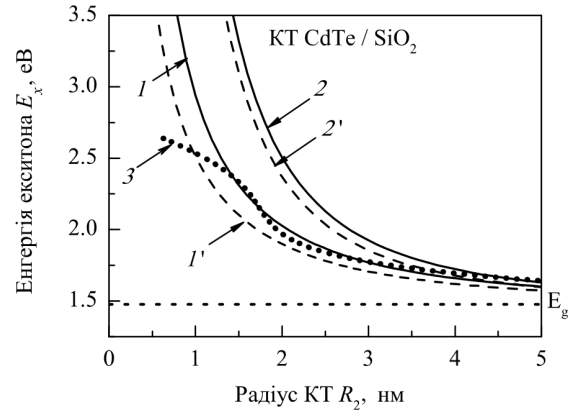
Рис. 2. Залежності енергії основного екситонного переходу E_x в КТ CdTe від радіуса КТ. Криві 1 і 1' відповідають скінченному бар'єру CdTe/SiO 2 , 2 і 2' – нескінченно високому бар'єру. Криві 1 і 2 побудовані з урахуванням змішування станів важких і легких дірок, 1' і 2' – враховано лише стан важкої дірки. Крива 3 – емпірична залежність енергії першого піка поглинання від радіуса КТ CdTe [20]
