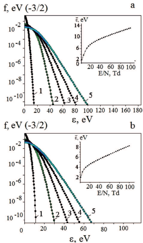
Рис. 1. Функції розподілу електронів за енергіями в розряді на суміші \text{HgI}_2\text{-Ne} = 0,54\text{-}99,46\% (а) і в суміші \text{HgI}_2\text{-Xe-Ne} = 0,64\text{-}9,03\text{-}90,33\% (b) для різних значень параметра E/N : 1 (1), 25,8 (2), 50,5 (3), 75,3 (4), 100 (5); в правій верхній частині рисунка наведена залежність середньої енергії електронів від параметра E/N
