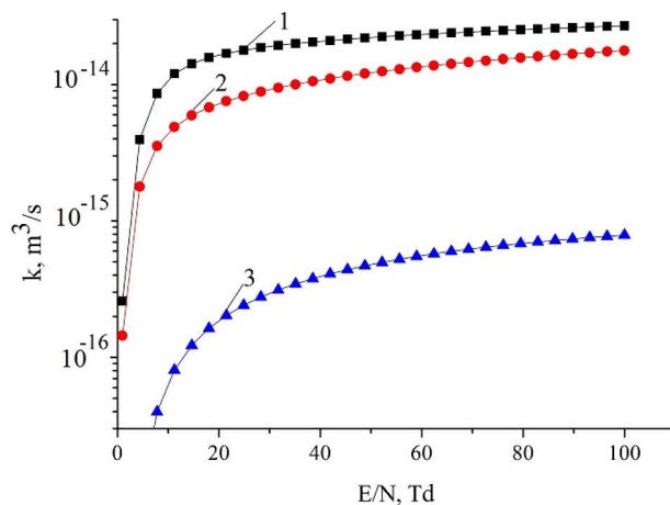
Рис. 3. Залежність констант швидкості дисоціативного збудження B^2\Sigma_{1/2}^+ -стану молекули моноїодиду ртуті електронами від параметра E/N в розряді у сумішах: \text{HgI}_2\text{-Ne} = 0,54\text{-}99,46\% (1) і \text{HgI}_2\text{-Xe-Ne} = 0,64\text{-}9,03\text{-}90,33\% (2), а також константи швидкості збудження метастабільного стану ^3P_2 атомів ксенону електронами
