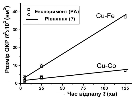
Рис. 5. Залежності розмірів ОКР R^3 від часу відпалу ПС Cu + Fe і Cu + Co при 600 °C
