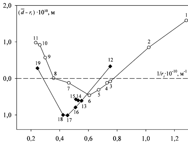
Рис. 6. Ізотерми (\bar{d} - r_i) - 1/r_i для однозарядних іонів у воді при 298,15 К
