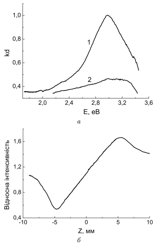
Рис. 4. Різницеві спектри поглинання (а) та спектр нормалізованого пропускання (б) відпаленого у повітрі зразка скла \text{Li}_2\text{B}_4\text{O}_7:\text{Gd,Ag} (спектри 1 і 2 – поглинання до і після видалення інтерфейсного шару, відповідно)
