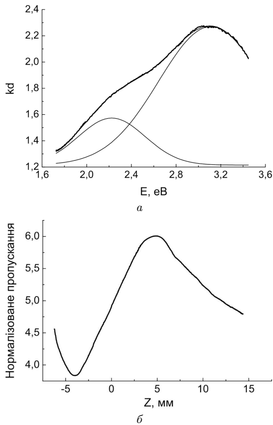
Рис. 3. Різницевий спектр поглинання з розкладом на складові (а) та спектр нормалізованого пропускання, отриманий з експериментального Z-scan спектра (б) для скла \text{Li}_2\text{B}_4\text{O}_7:\text{Gd,Ag} , відпаленого у вакуумі
