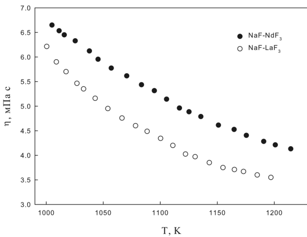
Рис. 1. Температурна залежність в'язкості розплавів NaF-LaF 3 та NaF-NdF 3
