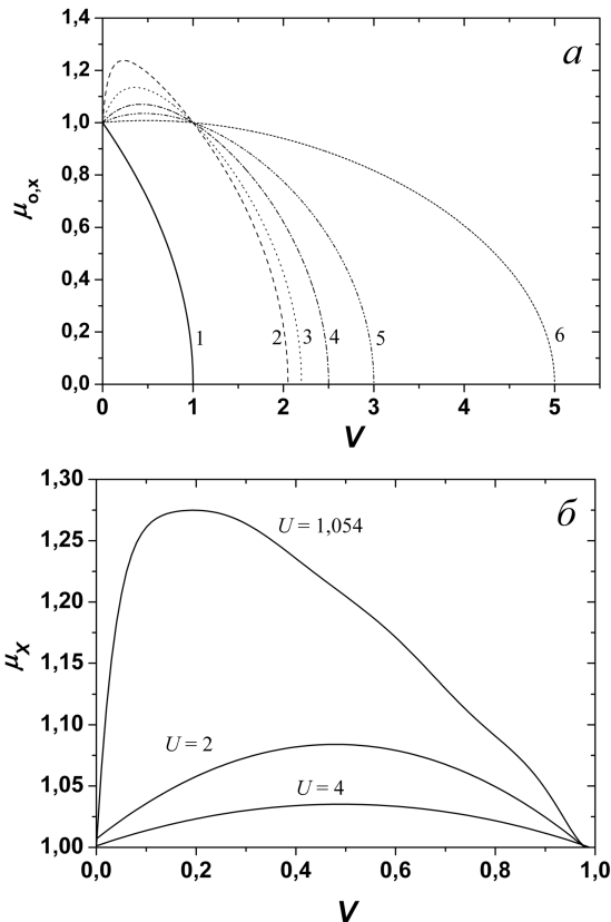
Рис. 1. Залежність коефіцієнта заломлення від V : a – звичайної хвилі (крива 1) і незвичайної хвилі при U = 1,1; 1,2; 1,5; 2; 4 (криві 2–6 відповідно), б – незвичайної хвилі при V від 0 до 1, U = 1,054; 2; 4
