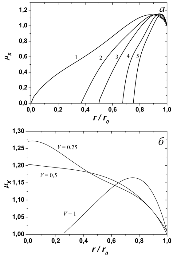
Рис. 2. Радіальна залежність \mu_x при зондуванні в перерізі У-ЗМ з внутрішнього боку (більшого магнітного поля) B_0 = 0,72 Т, зондуюча частота f_0 = 18 ГГц і N(r) = N_0[1 - (r/r_0)^2] , де N_0 – густина плазми на магнітній осі, r_0 = 19 см – відстань від магнітної осі до краю плазми; a – криві 1, 2, 3, 4, 5 відповідають V_0 = 2; 3; 3,5; 4; 5 , б – V_0 = 0,25; 0,5; 1
