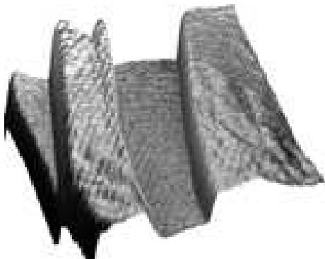
Рис. 1. 3D-вид морфології свіжосколотої поверхні кристала \text{CdI}_2 після відривання площини за допомогою скотчу (image size: 20 \times 20 мкм; z range: 24,40 нм)
