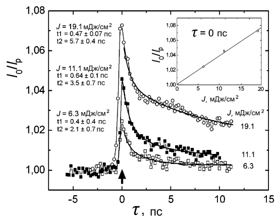
Рис. 2. Залежності I_0/I_p від \tau при густинах енергії збуджуючого імпульсу J = 6,3 ; 11,1 і 19,1 мДж/см 2 . На вставці показано залежність I_0/I_p від J при \tau = 0 пс. Довжини хвиль зондуючого світла 680–690 нм
