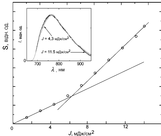
Рис. 1. Нормовані спектри ФЛ нано-Si/SiO 2 при густині енергії збуджуючого імпульсу J = 4,3 мДж/см 2 і 11,5 мДж/см 2 (див. вставку) і люкс-інтенсивностна характеристика S(J) . Зміна нахилу залежності S(J) спостерігається при J = 6 мДж/см 2
