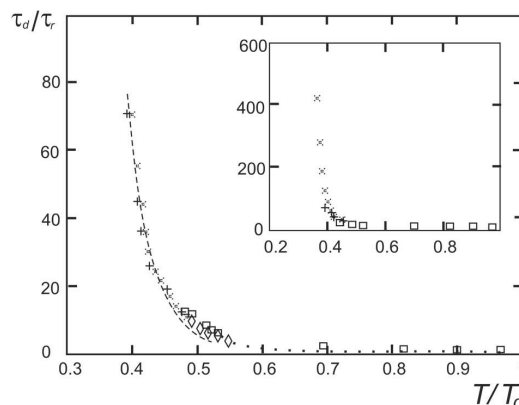
Рис. 6. Температурна залежність відношення \tau_d(t) = \tau_d(t)/\tau_r , де береться з робіт: + – з [25], \square – з [29], \times – з [30], \diamond – з [31]. Точками представлені інтерполяційні значення
