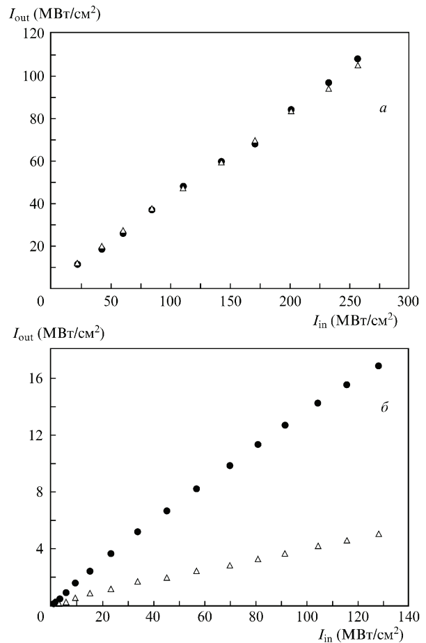
Рис. 1. Залежність інтенсивності випромінювання, що пройшло через зразок, від інтенсивності падаючого випромінювання для аморфного і 100% кристалічного зразка при а – \lambda = 1064 нм і б – \lambda = 532 нм: ● – аморфний зразок, \Delta – повністю кристалічний зразок ЗС
